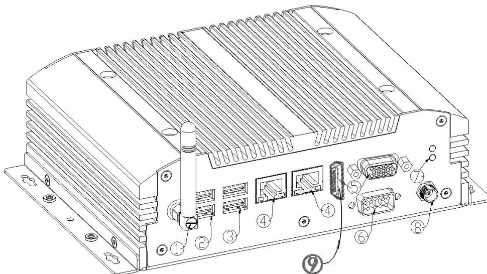
图 2: 后面板
